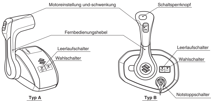
FERNBEDIENUNGSGEHÄUSE (OPTION)
