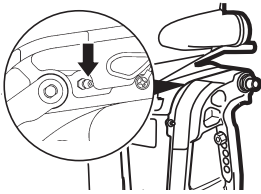
Drehgelenkkonsole
