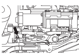
Alavanca de embreagem
