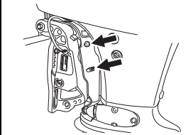
DF115BG Tableau arrière L
