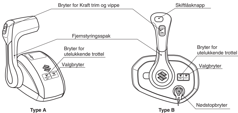
FJERYSTRINGSBOKS (EKSTRAUTSTYR)
