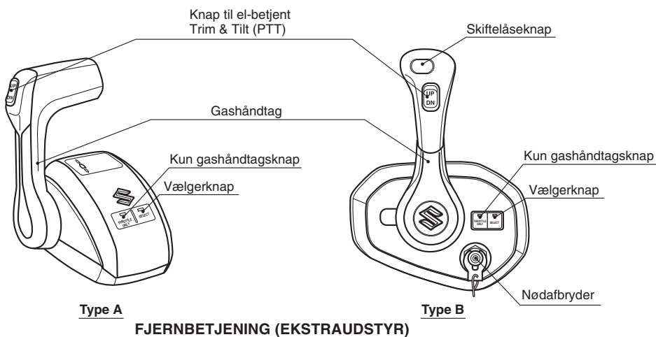
FJERNBETJENING (EKSTRAUDSTYR)
