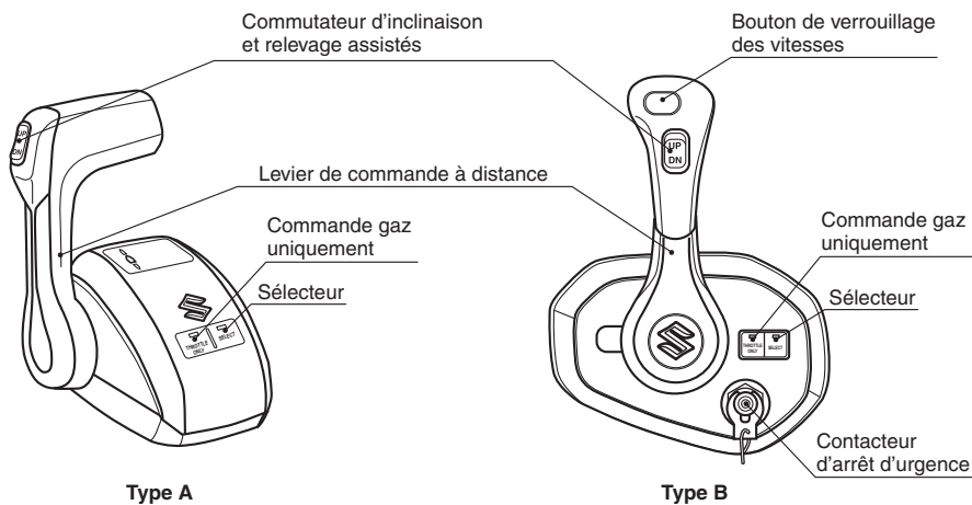
BOÎTIER DE COMMANDE À DISTANCE (OPTION)
